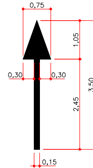
SIGA EM FRENTE (SETA: H=3,50m)
