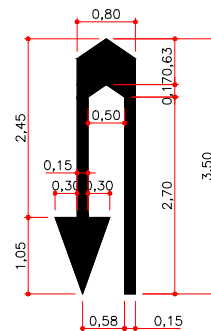
SETA INDICATIVA DE RETORNO NA VIA (SETA: H=3,50m)
