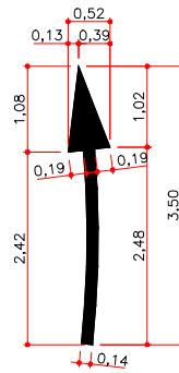
SETA INDICATIVA DE MOVIMENTO EM CURVA (SETA: H=3,50m)
