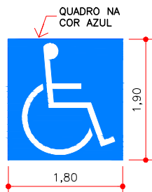
SÍMBOLO NO PAVIMENTO
