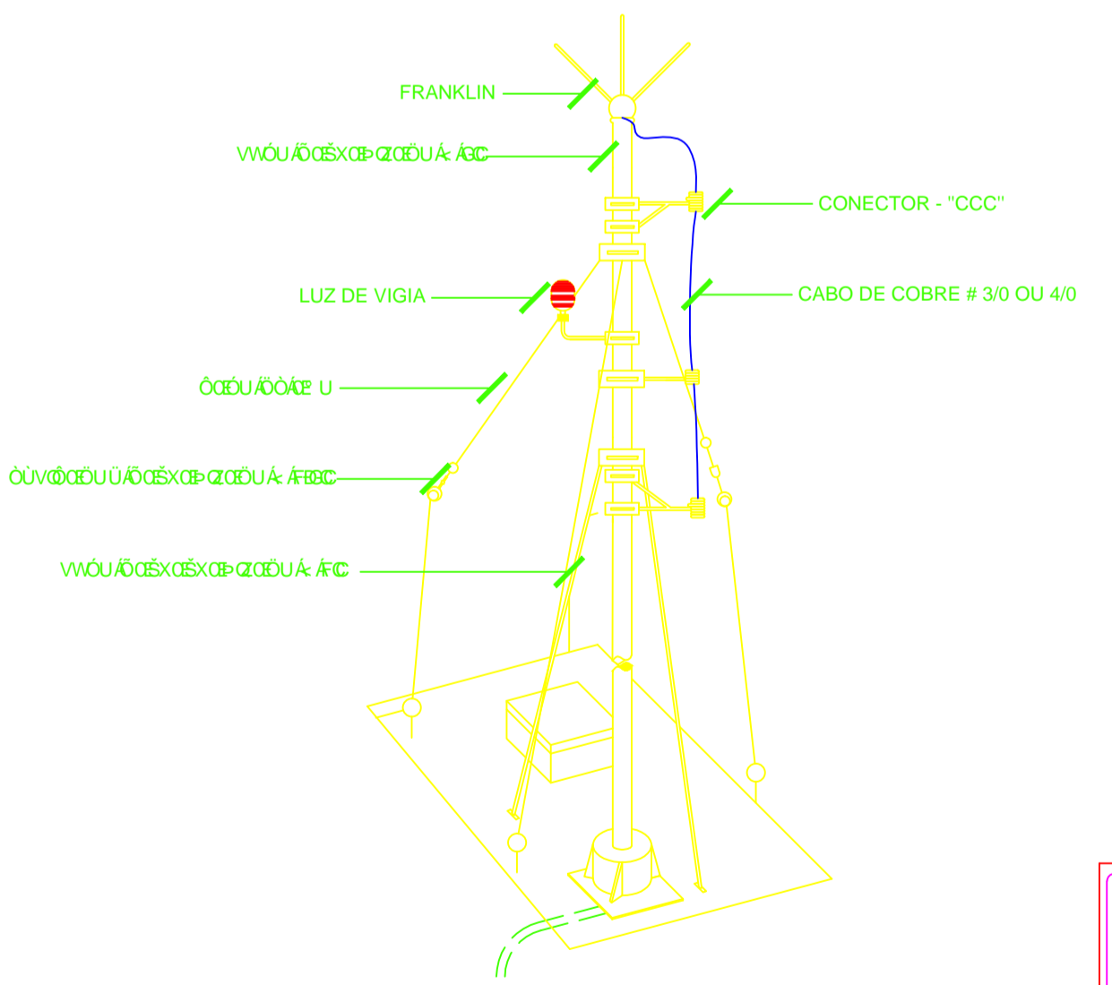
FRANKLIN CONECTOR "CCC" CABO DE COBRE # 3/0 OU 4/0 LUZ DE VIGIA
