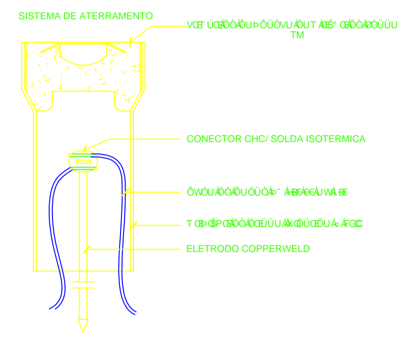
SISTEMA DE ATERRAMENTO
