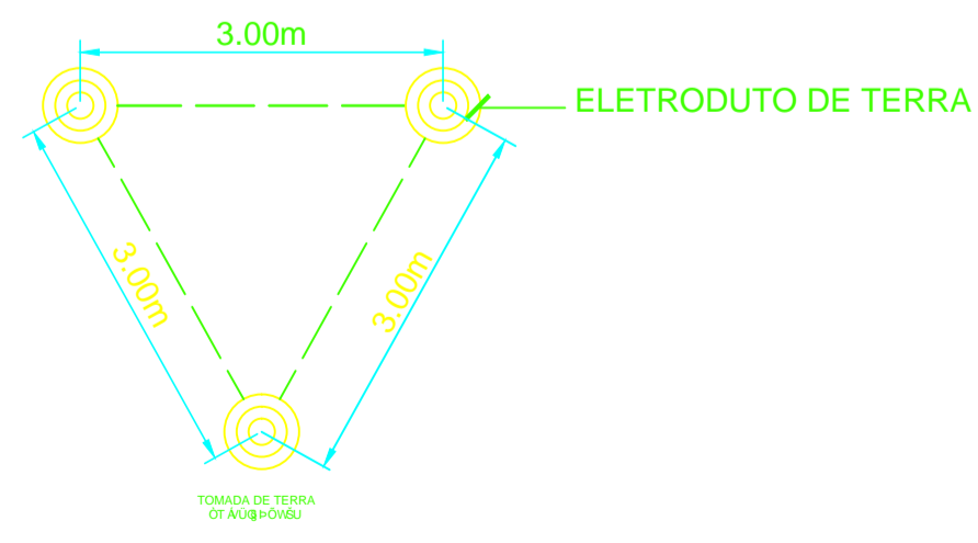
NOTA: PARA ELETRODOS DE 3.00m DE COMPRIMENTO O ESPAÇAMENTO DEVE SER 3.00m
