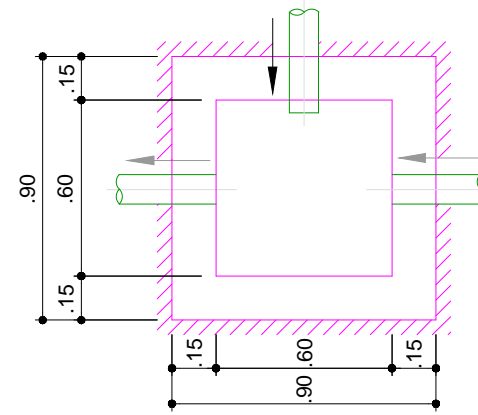
PLANTA BAIXA SEM ESCALA
