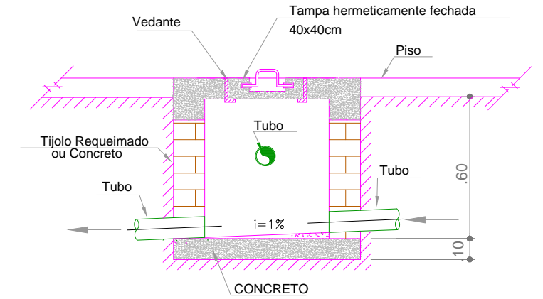
CORTE SEM ESCALA
