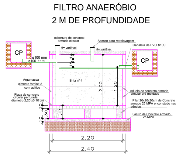
CORTE FITRO ANAERÓBIO
