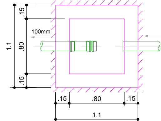
PLANTA BAIXA SEM ESCALA
