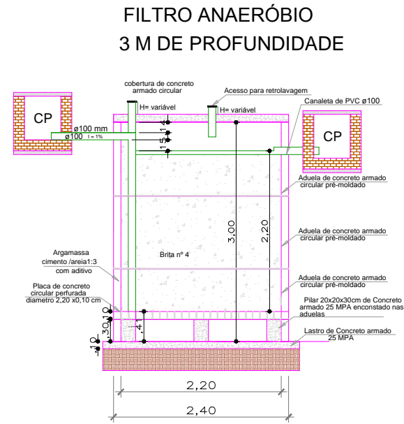
CORTE FITRO ANAERÓBIO
