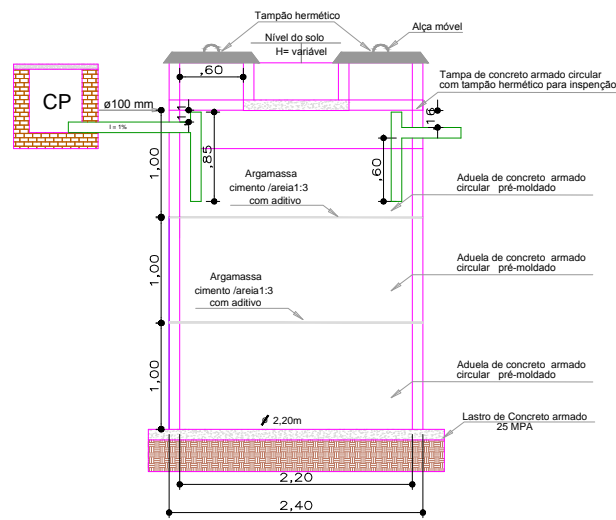
CORTE TANQUE SÉPTICO
