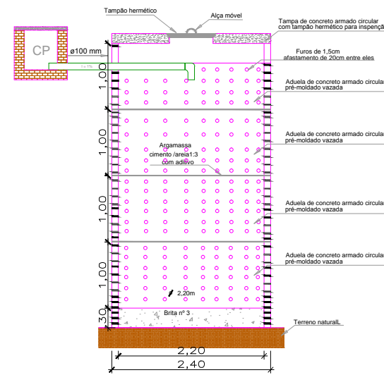
CORTE
