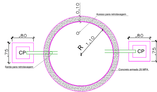
PLANTA BAIXA
