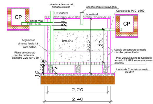
CORTE
