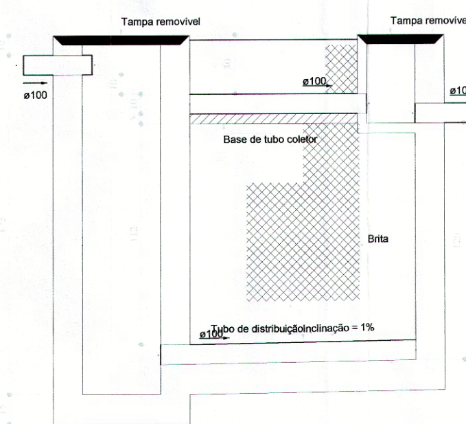
Filtro anaeróbio Corte 1 - ESC. 1:25
