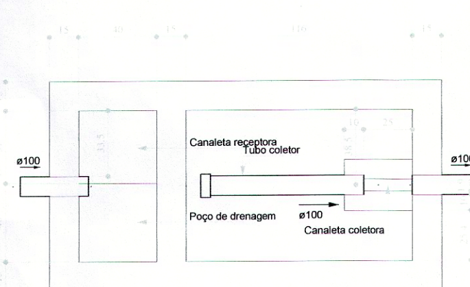
Filtro anaeróbio Planta baixa - ESC. 1:25
