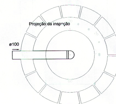
Sumidouro Planta baixa - ESC. 1:25
