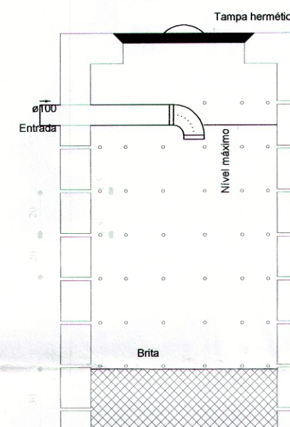
Sumidouro Corte 1 - ESC. 1:25
