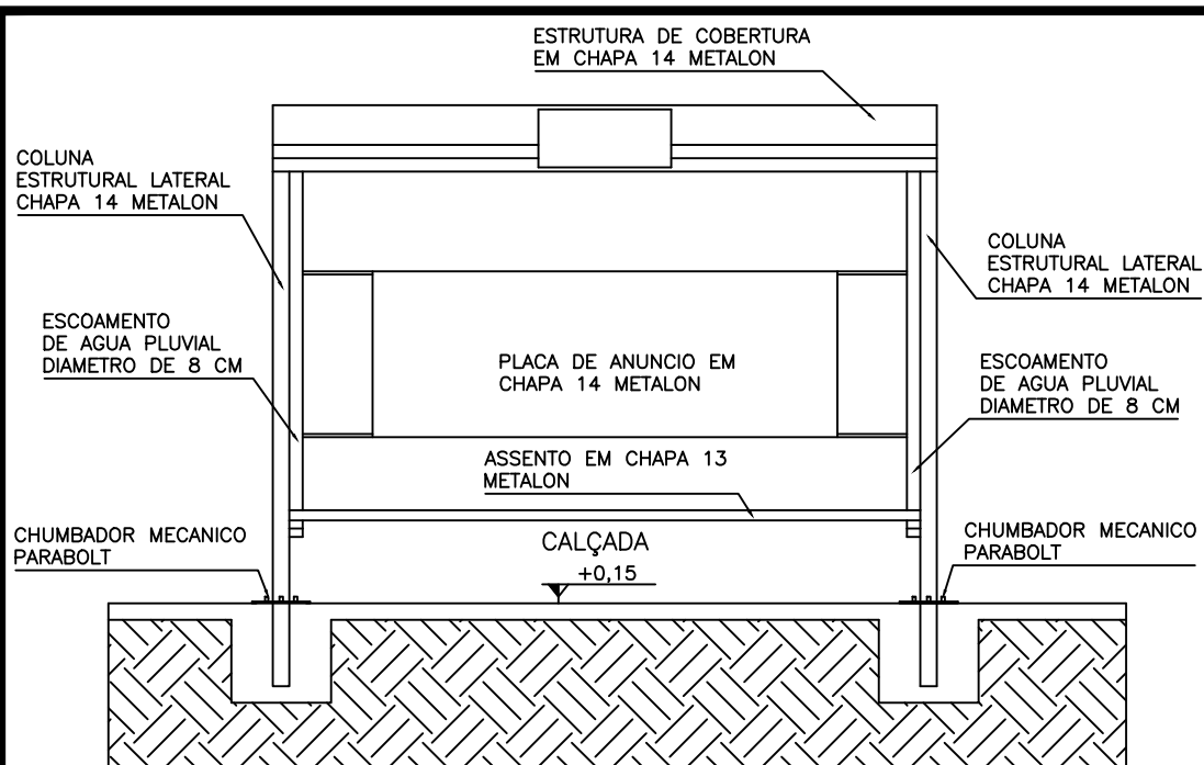
1 DETALHAMENTO 01 Escala 1:50
