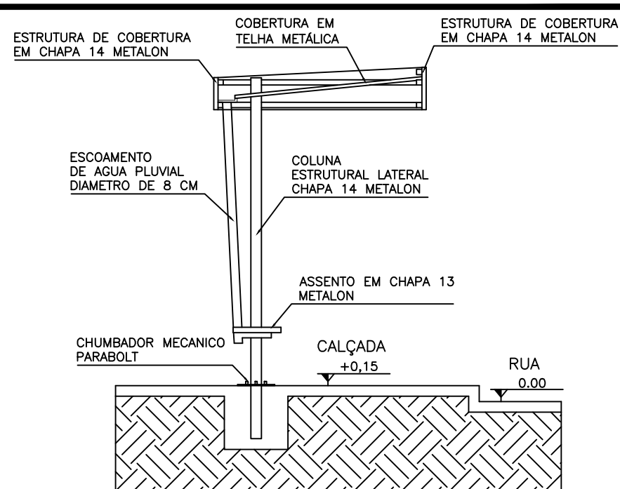
3 DETALHAMENTO 03 Escala 1:50
