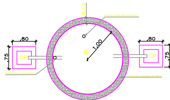
PLANTA BAIXA
