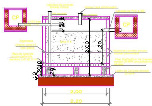
CORTE FITRO ANAERÓBIO
