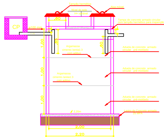
CORTE TANQUE SÉPTICO
