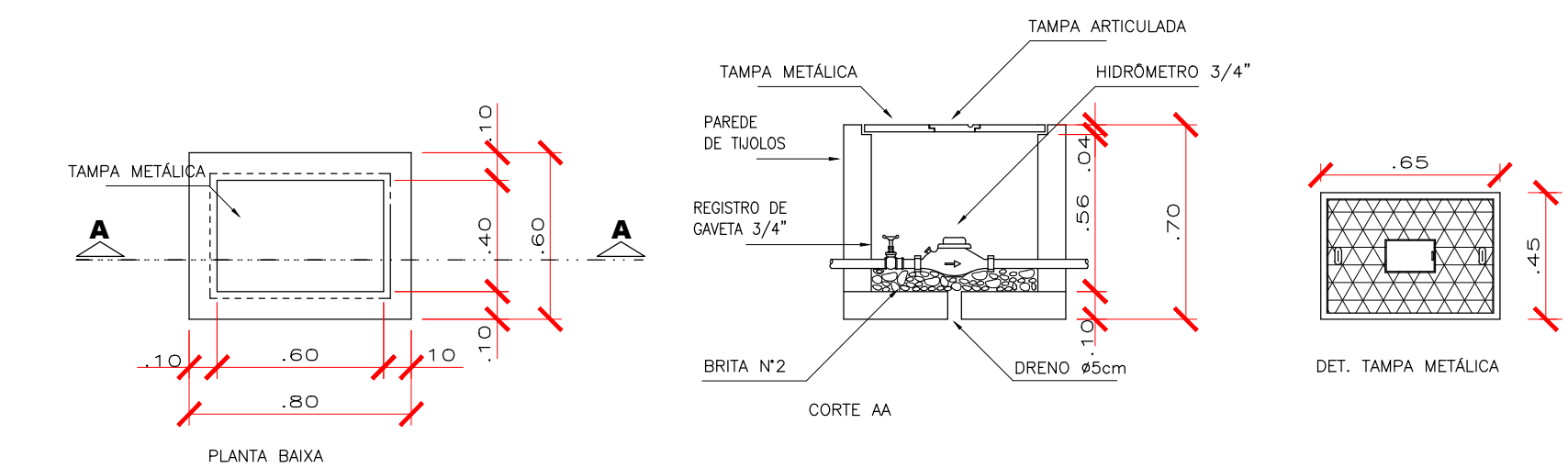
02 DETALHE ABRIGO/ CAIXA HIDRÔMETRO Esc: 1/25
