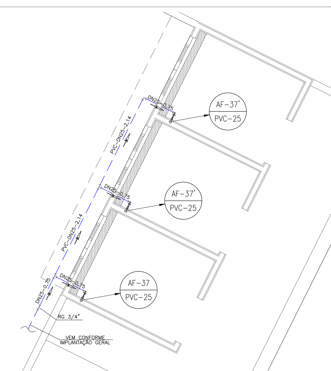
03 PLANTA BAIXA - ABRIGO DE RESÍDUOS SÓLIDOS Esc: 1/50
