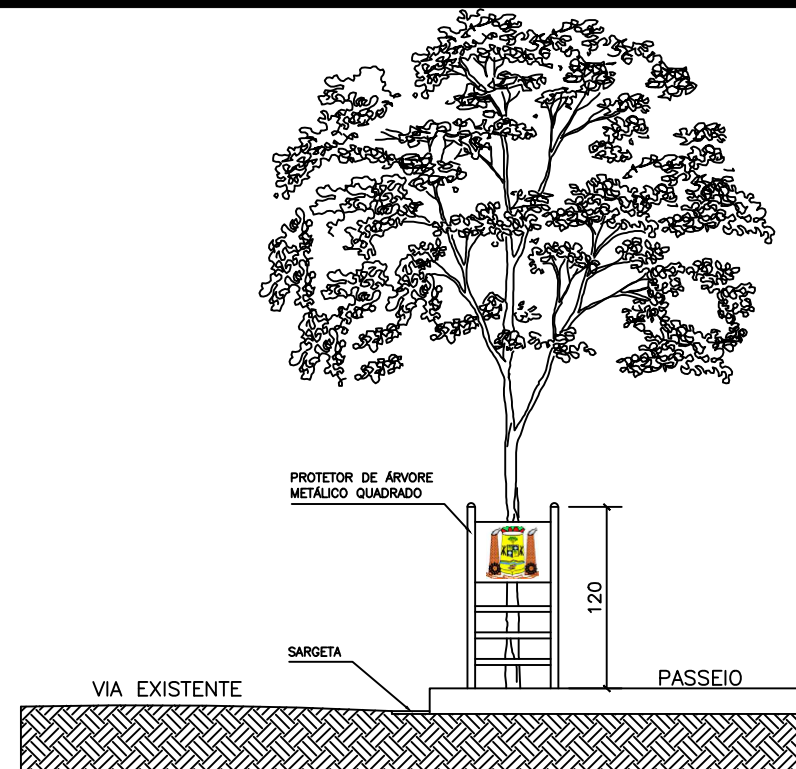
② VISTA 02 1:50
