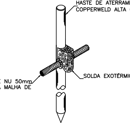
DETALHE 13
