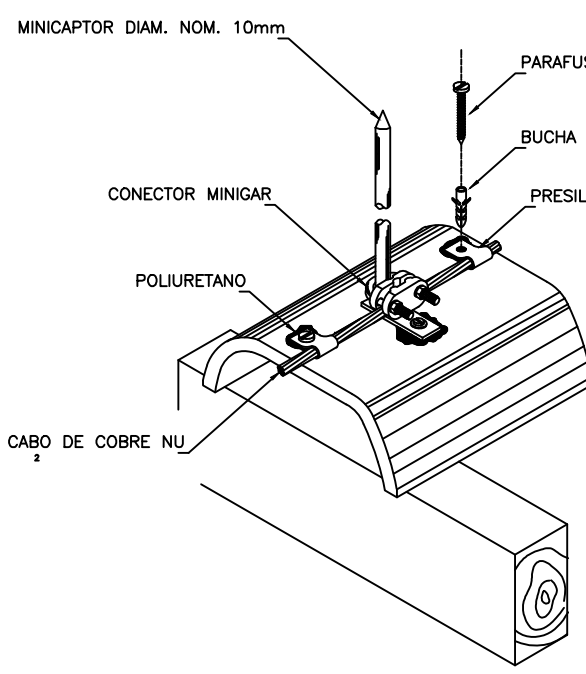
DETALHE 5
