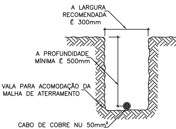
DETALHE 11
