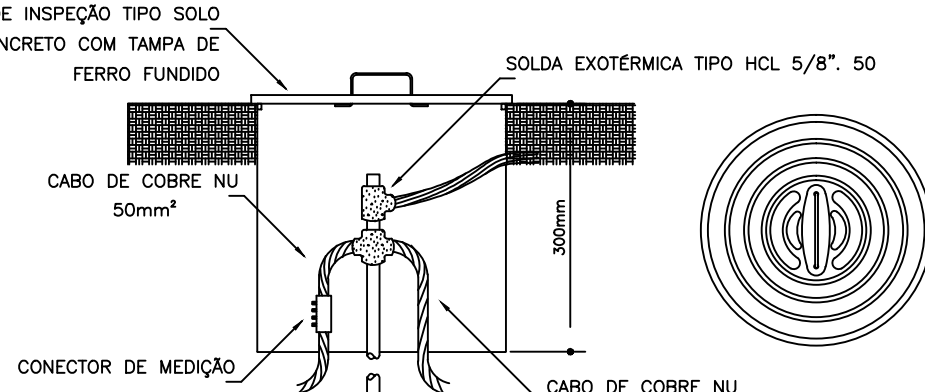
DETALHE 14
