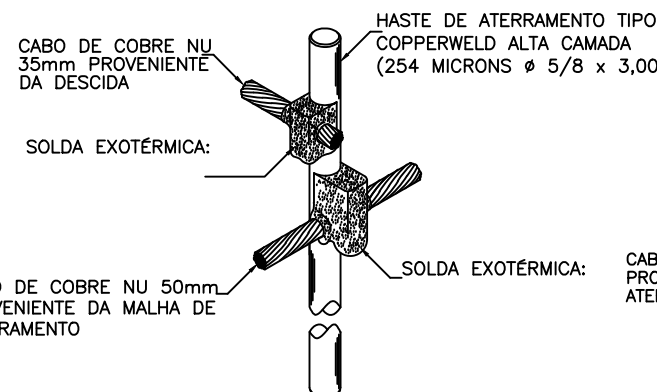
DETALHE 12
