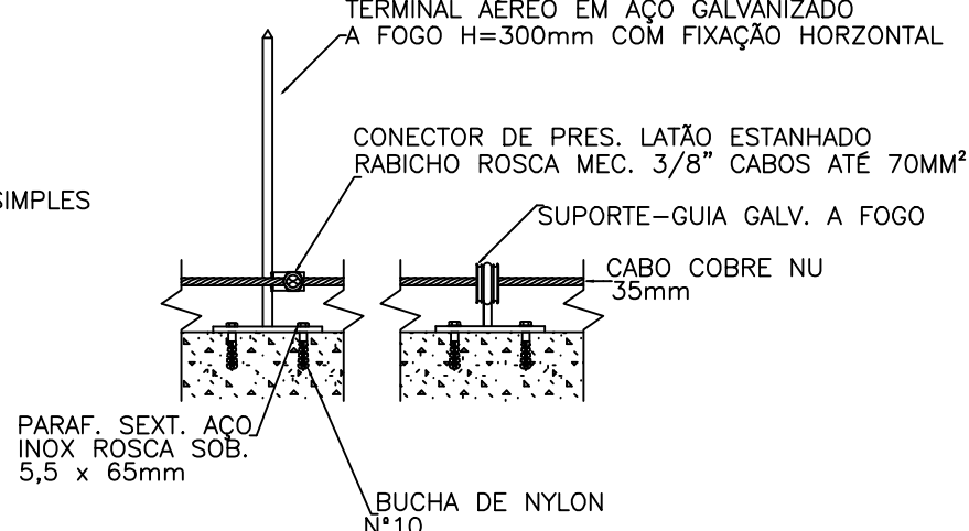
DETALHE 8
