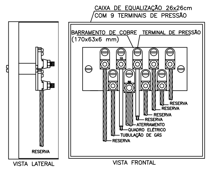
DETALHE 10
