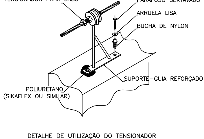
DETALHE 9
