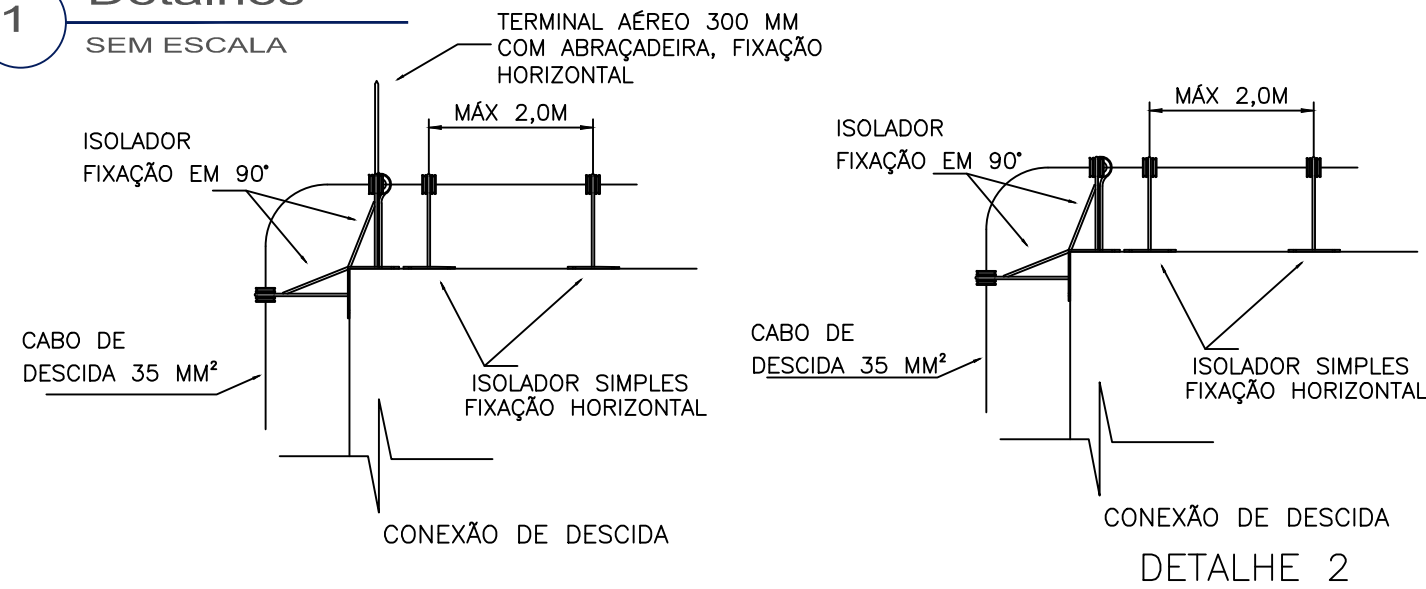
DETALHE 2
