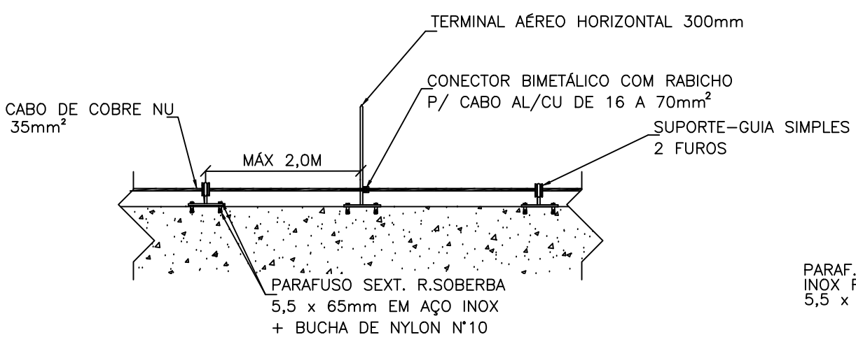
DETALHE 7
