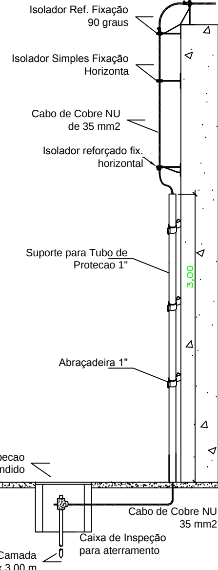
DETALHE 17
