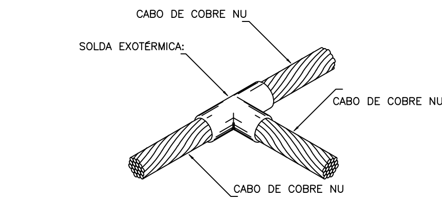
DETALHE 15
