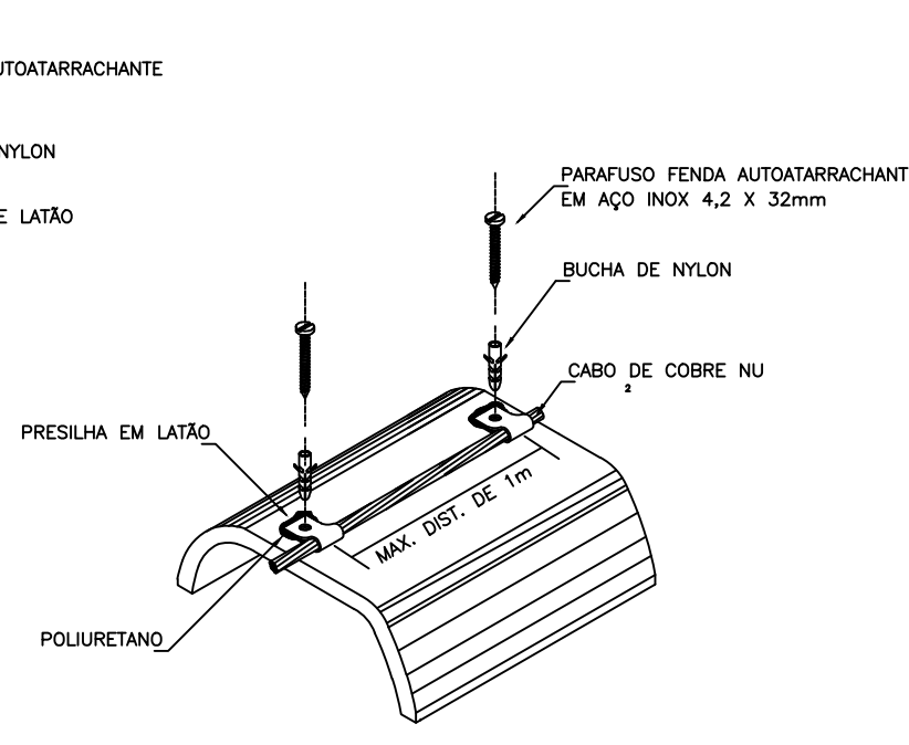
DETALHE 6
