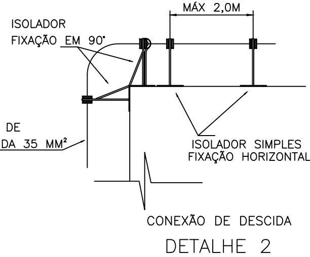
DETALHE 2
