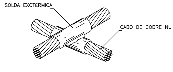
DETALHE 16
