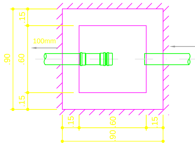
PLANTA BAIXA SEM ESCALA
