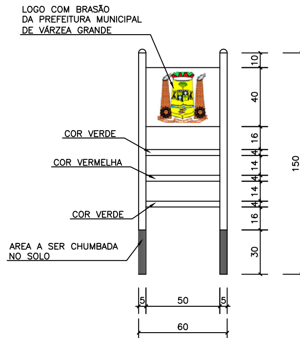
2 DETALHAMENTO 01 1:20
