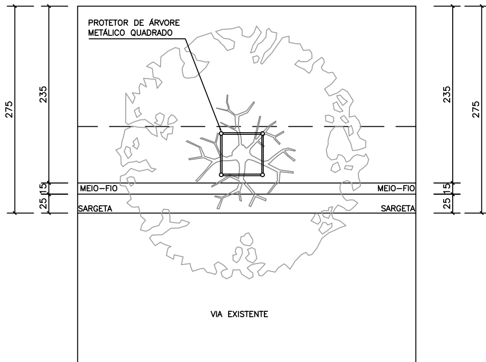
1 PLANTA BAIXA 1:50
