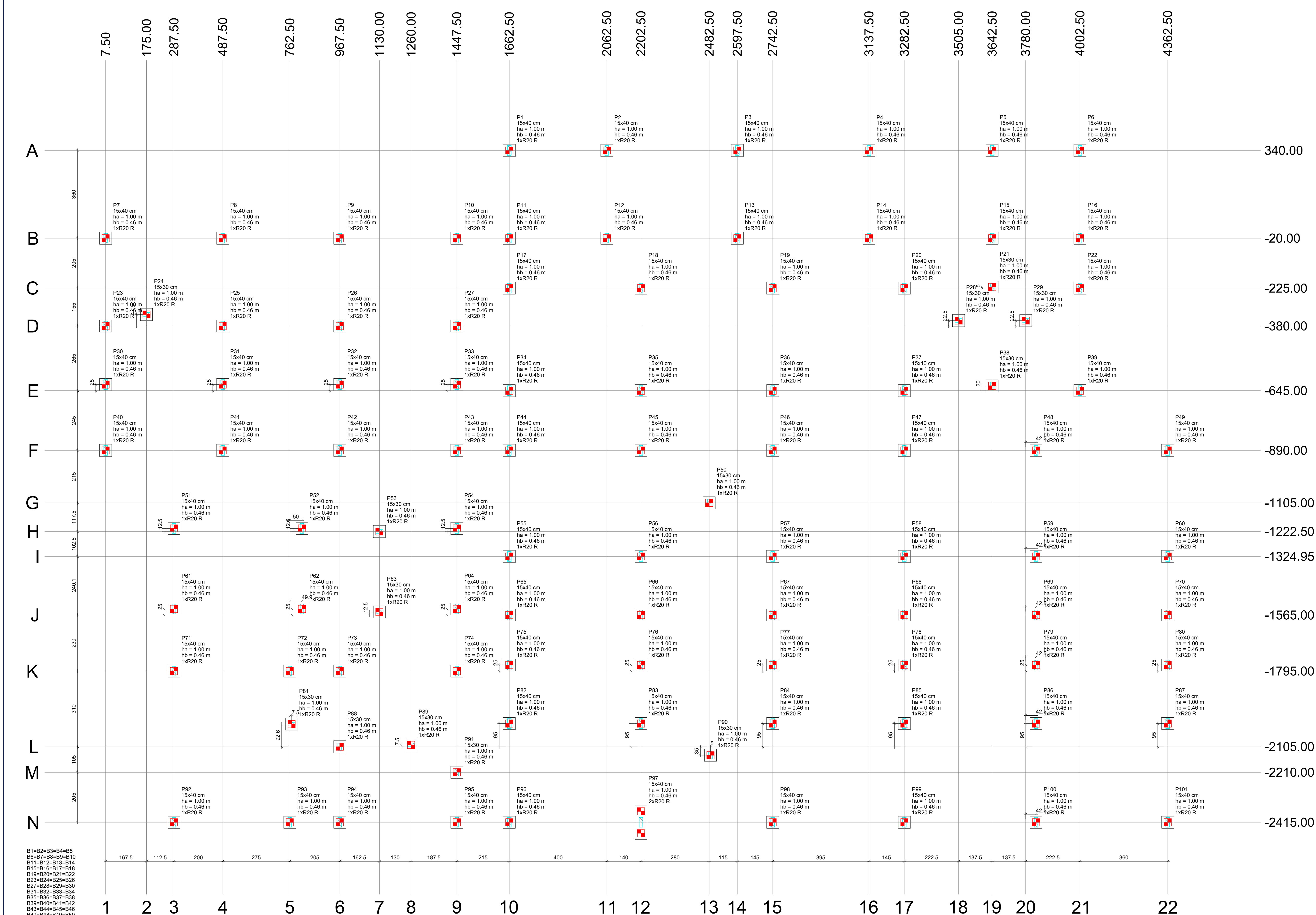
Planta de locação escala 1:25
