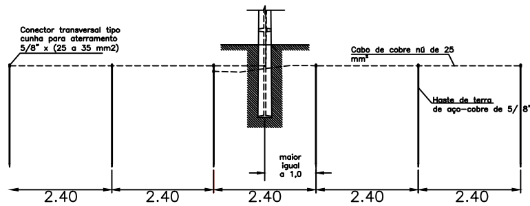
DETALHE MALHA DE ATERRAMENTO
